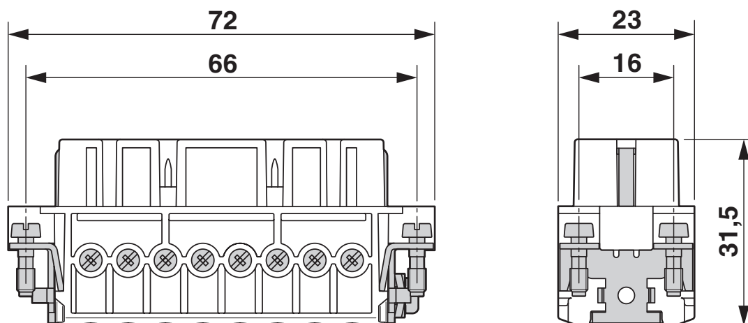
Dessin coté
