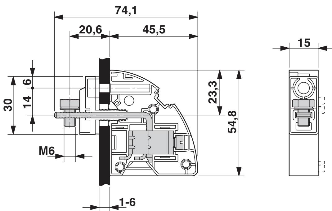
Dessin coté
