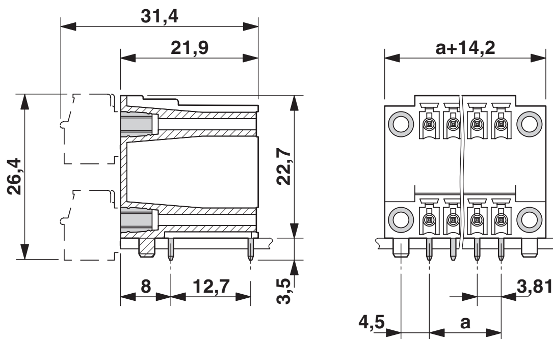
Dessin coté
