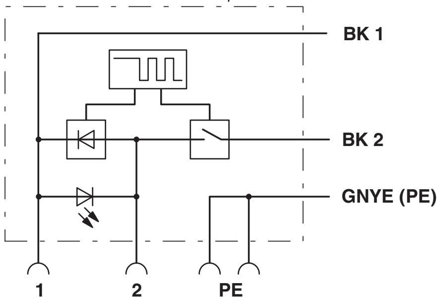
Schaltplan
