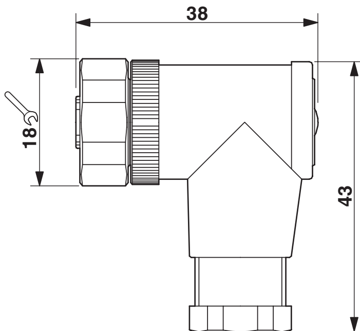
Maßzeichnung
