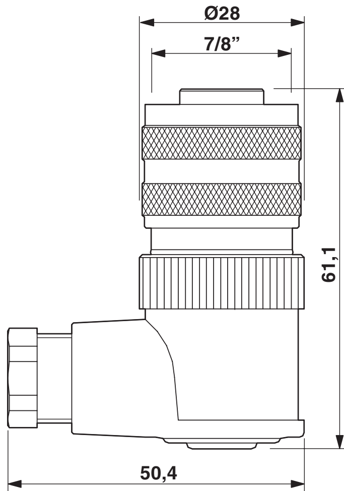
Maßzeichnung
