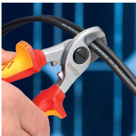
Taglio del cavo con cesole per cavo: taglio facile, pulito, senza deformazione del cavo
