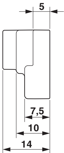
Esquema de dimensiones
