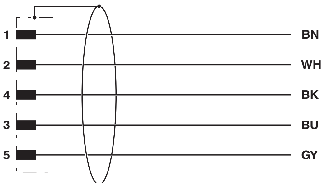
Diagrama eléctrico
