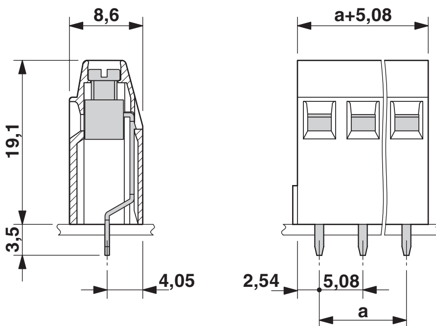
Maßzeichnung
