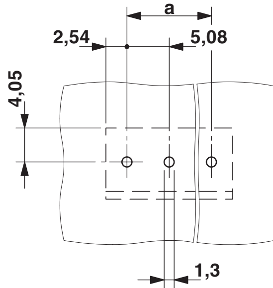
Bohrplan/Lötpadgeometrie
