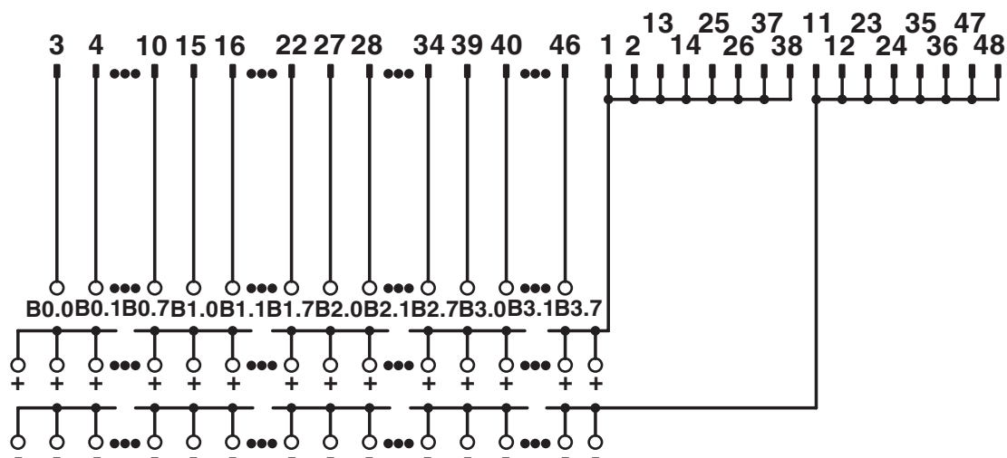
Schéma des connexions FFLKMS 50/32IM/PLC
