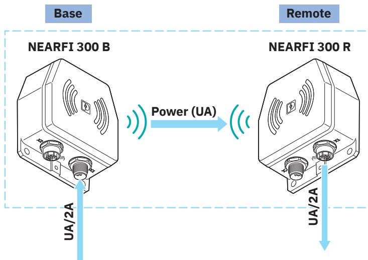
Plano esquemático
