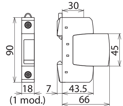
Maßbild DG SU 1P 120
