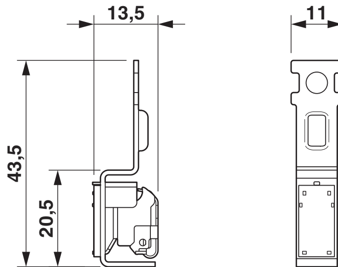
Maßzeichnung
