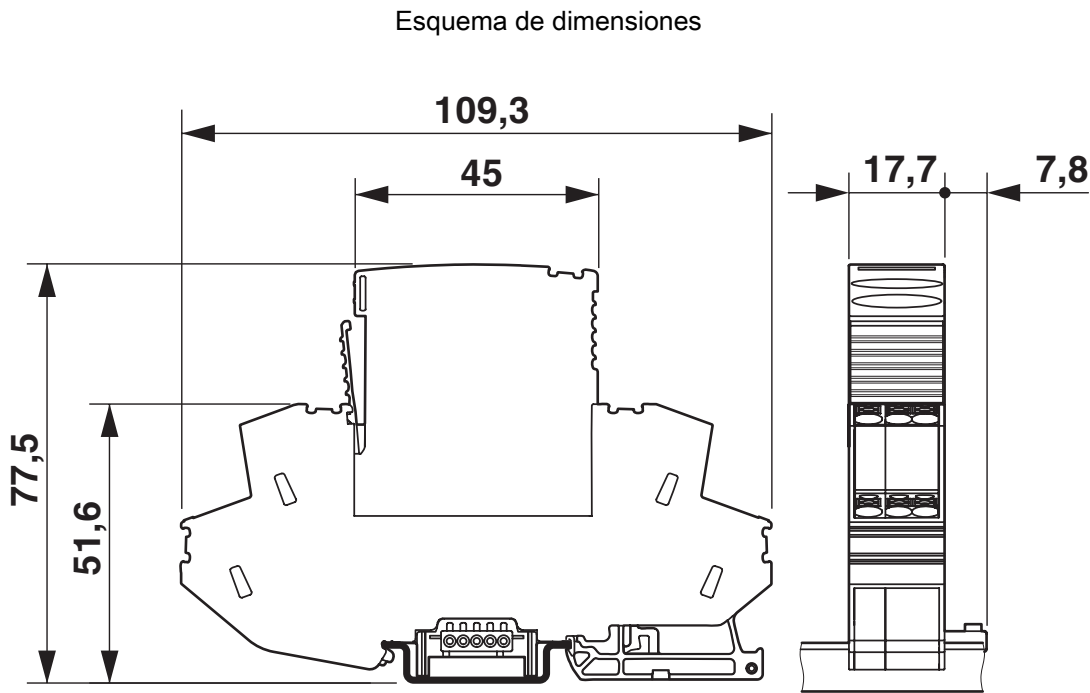
Plano esquemático
