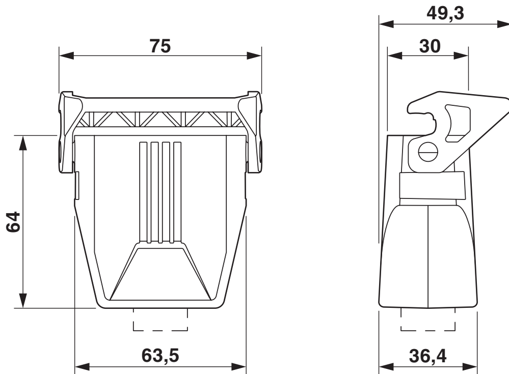
Maßzeichnung
