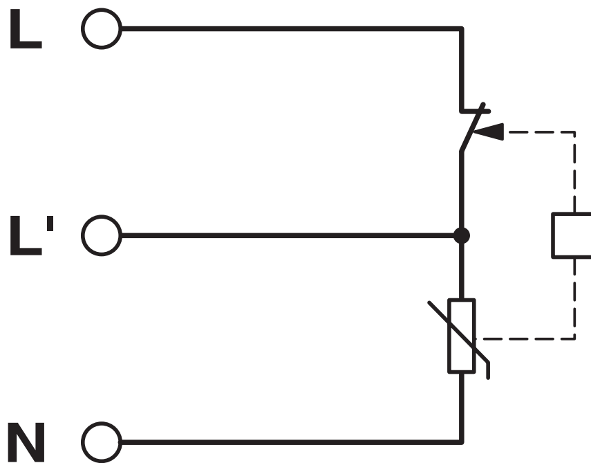
Schaltplan
