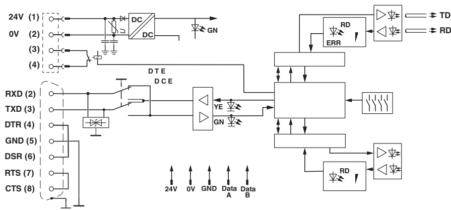
Schéma fonctionnel
