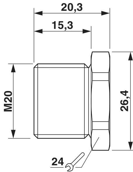
Maßzeichnung
