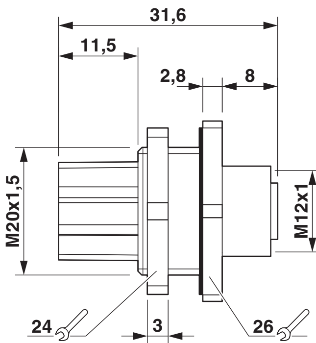
Maßzeichnung
