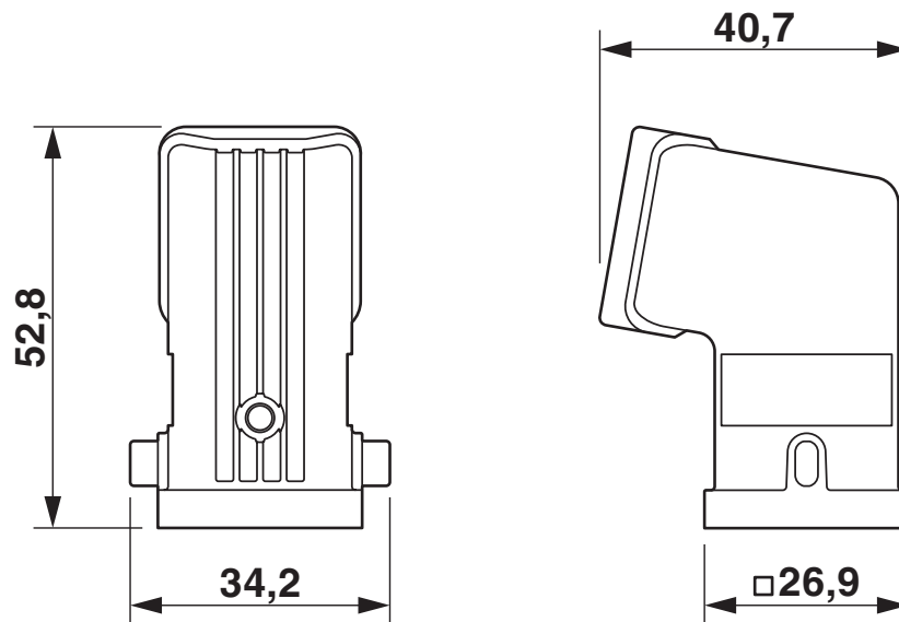
Maßzeichnung
