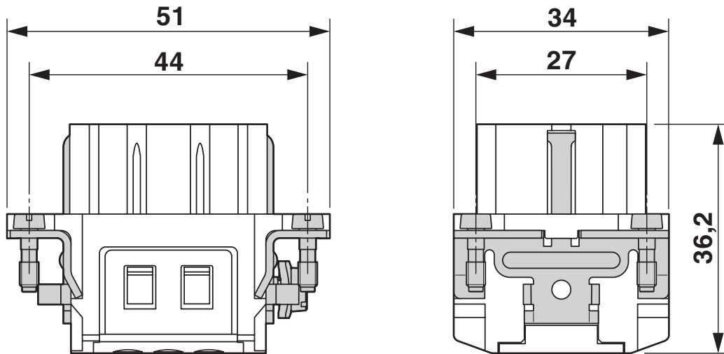
Maßzeichnung
