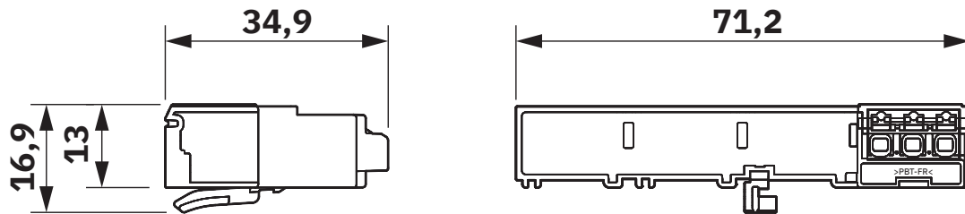
Maßzeichnung
