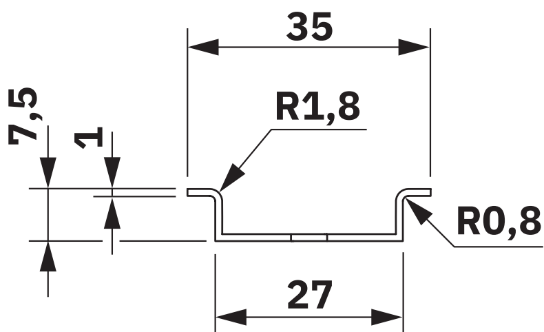
Dessin coté
