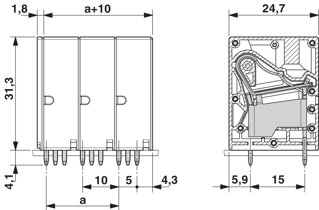
Dessin coté
