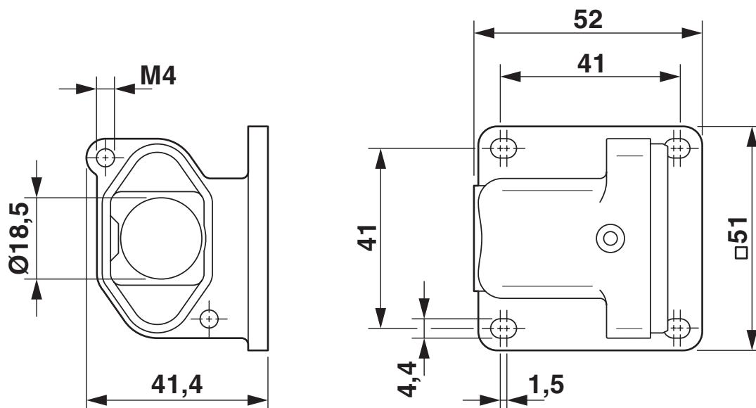
Dessin coté
