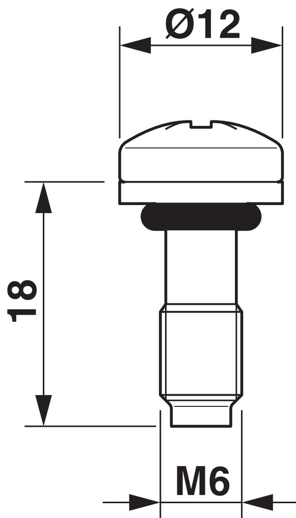
Dessin coté
