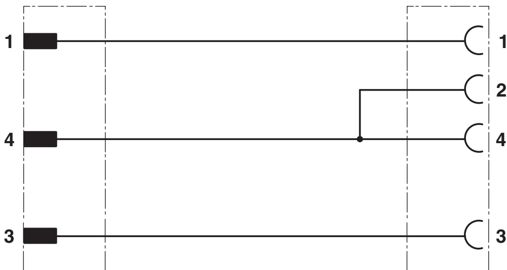
Diagrama eléctrico
