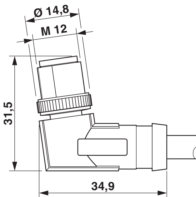
Dessin coté
