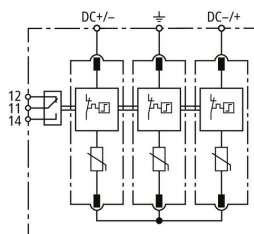
Schema di principio DG M YPV 1200 FM - old
