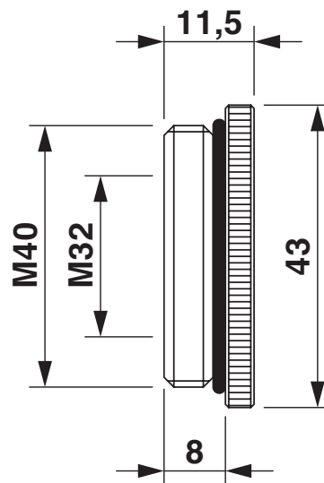
Maßzeichnung
