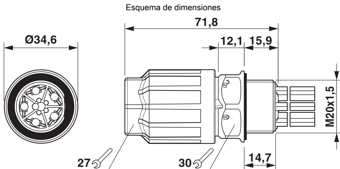
Dibujo acotado de QPD W 5 x 2,5 M20
