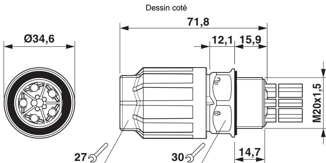
Dessin coté QPD W 5x2,5 M20
