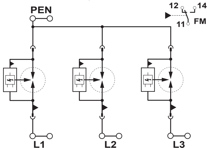
Diagrama eléctrico
