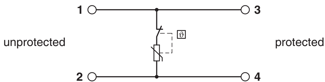
Diagrama eléctrico
