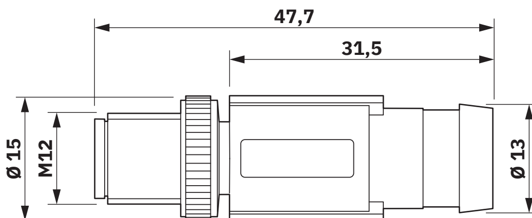
Dessin coté
