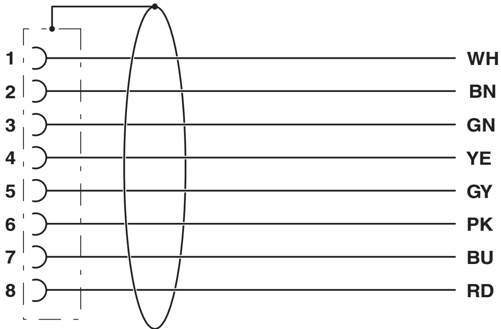
Diagrama eléctrico
