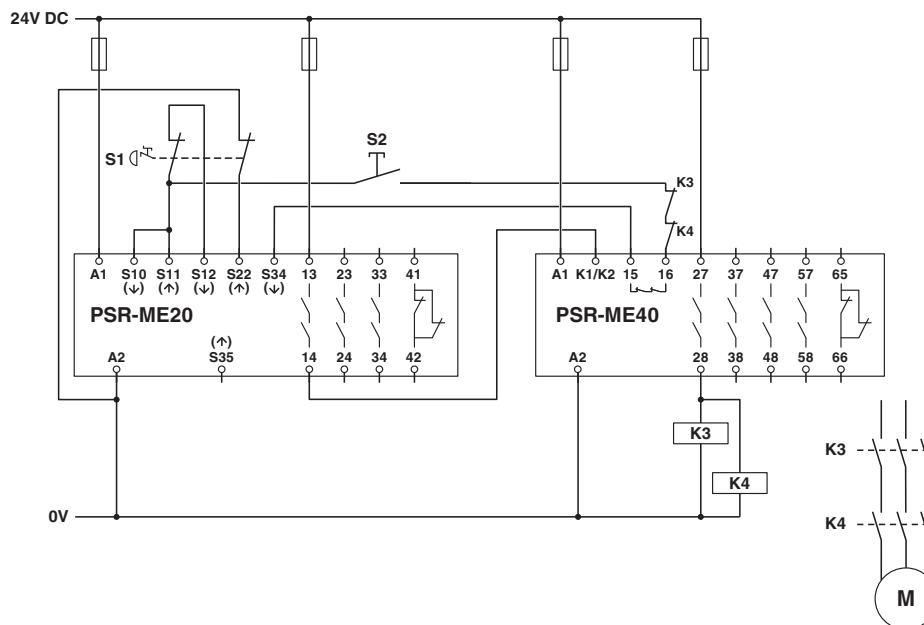
Diagrama eléctrico
