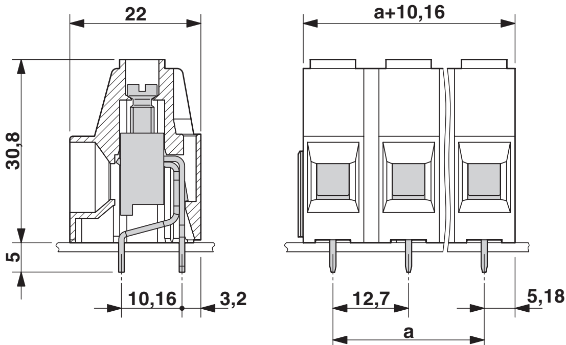
Maßzeichnung
