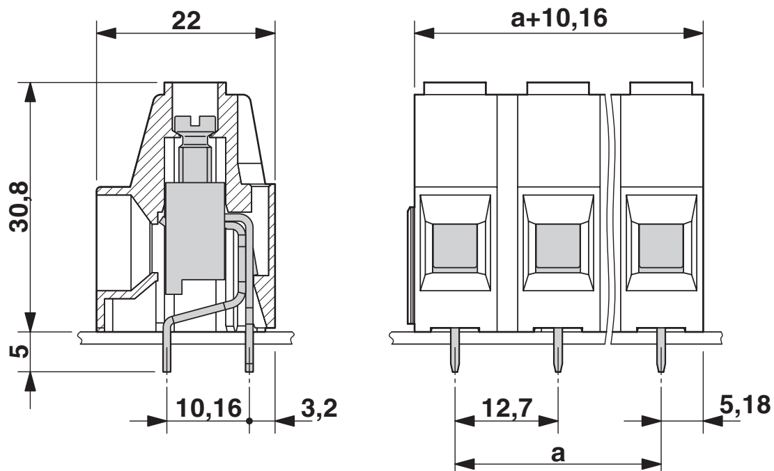
Dessin coté
