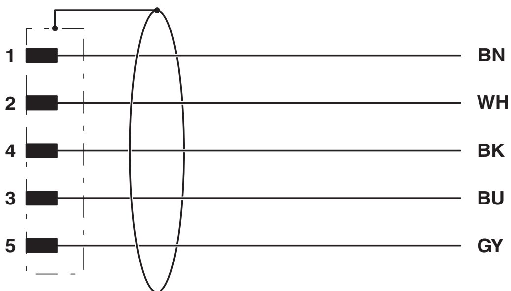
Diagrama eléctrico
