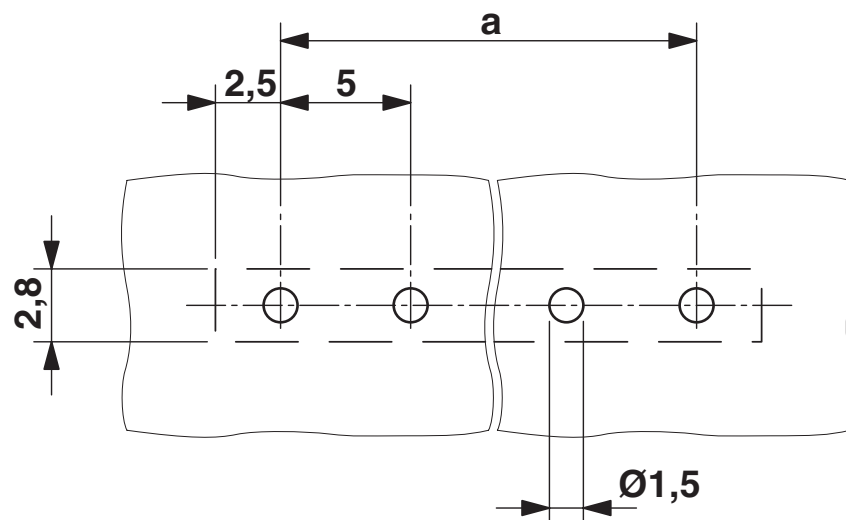
Esquema de taladros/geometría pads soldadura
