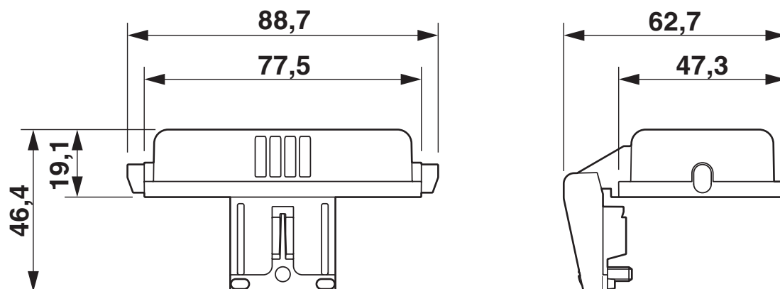
Dessin coté
