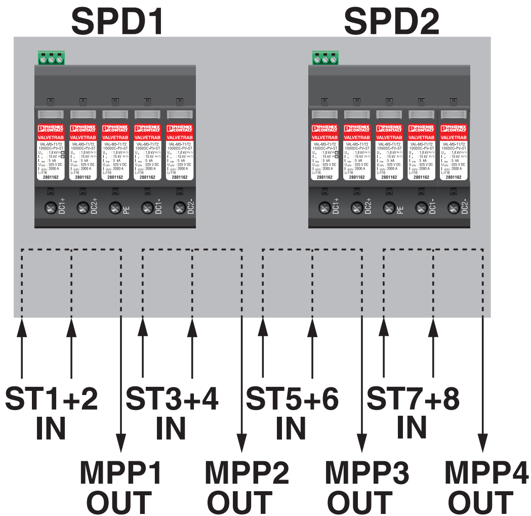
Schematische Applikationszeichnung
