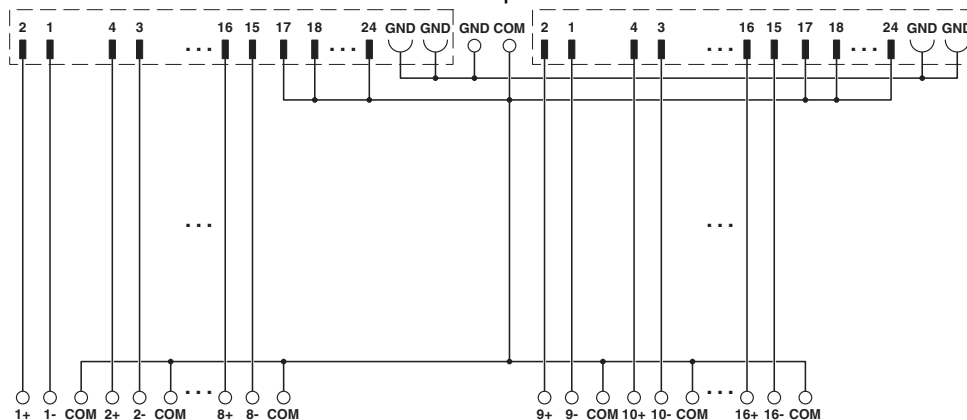
Schaltplan
