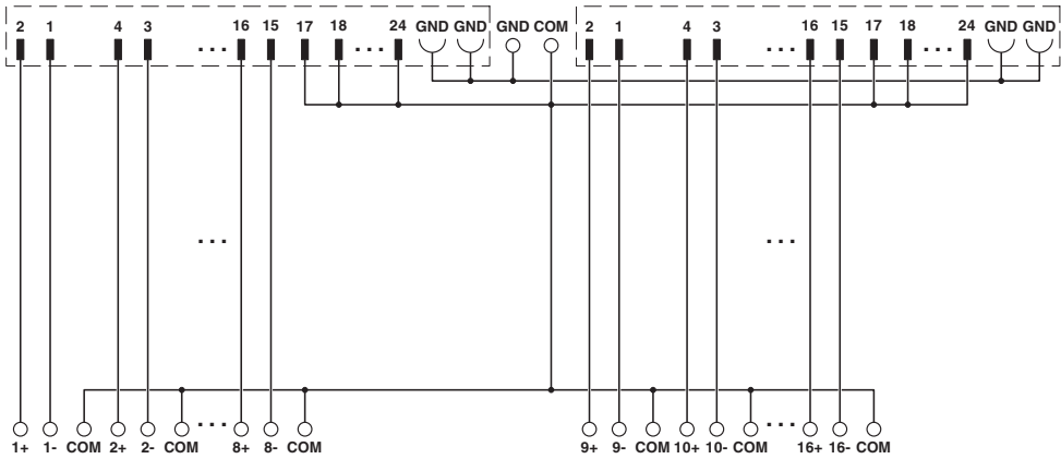
Diagrama eléctrico
