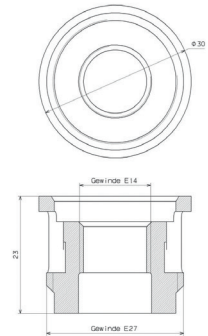
Maßbild RED E27 E14 ÜGK MB
