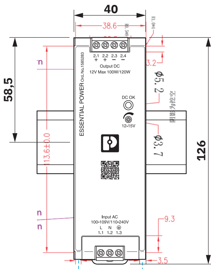
Maßzeichnung
