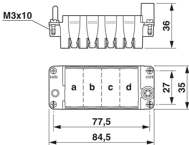
Dessin coté
