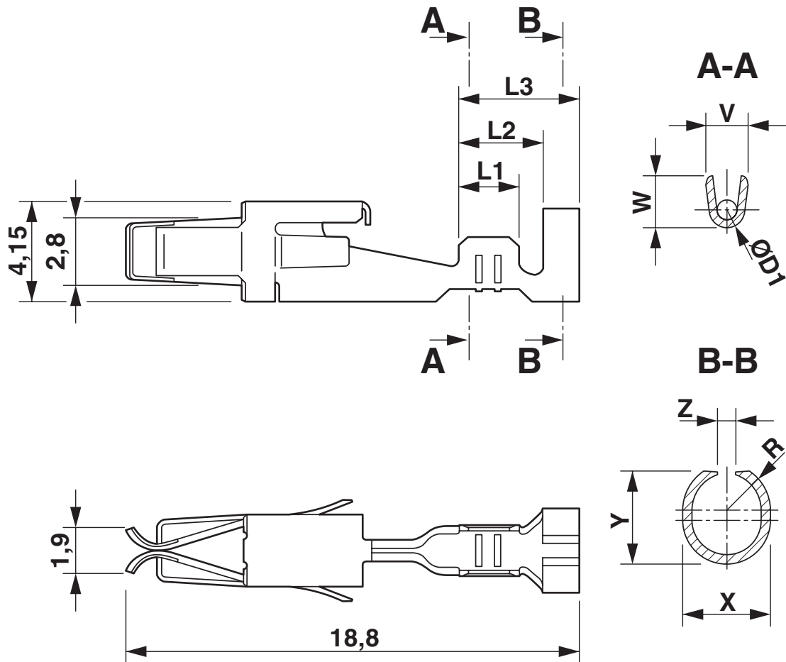
Dessin coté
